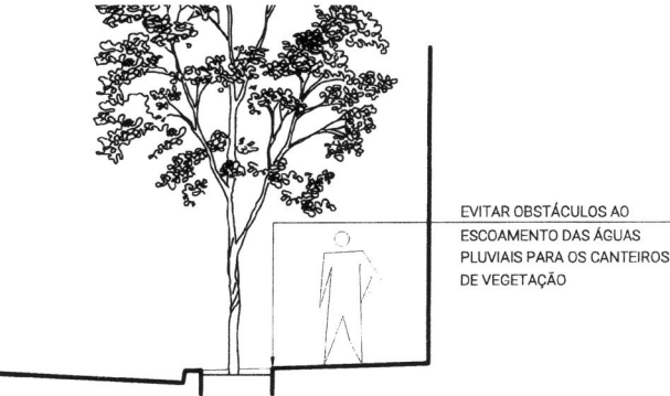
CORTE
